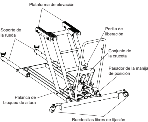
Figura 1: nomenclatura de los modelos T-1250
