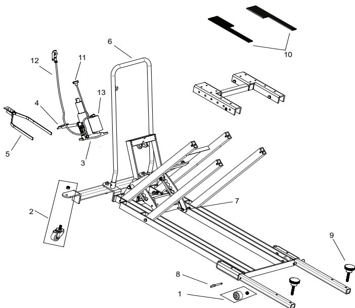
Figura 5: ilustración de piezas de repuesto para el modelo T-1250
