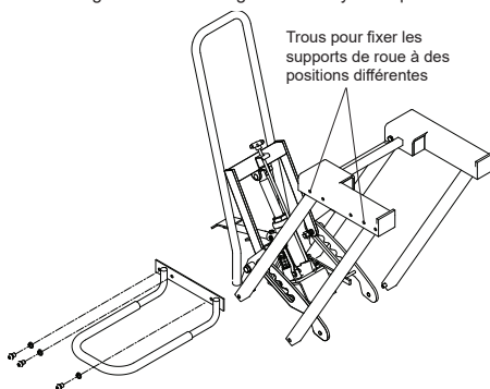
Figure 3 : Assemblage des supports de roue
