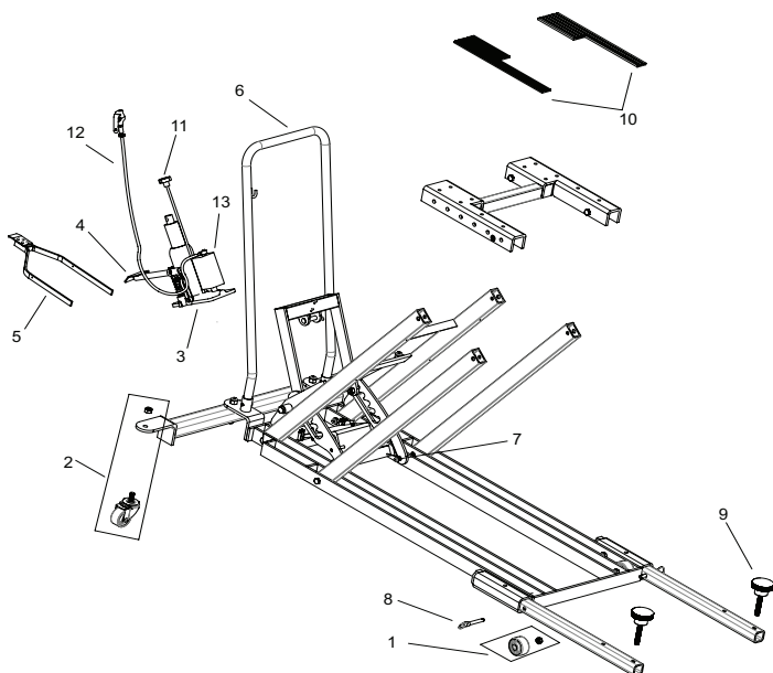
Figure 5 : Illustration des pièces de rechange du modèle T-1250
