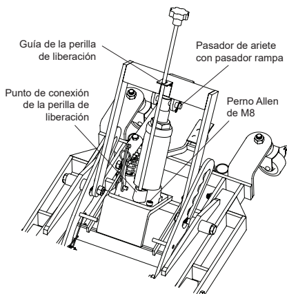
Figura 2: conjunto de la unidad hidráulica
