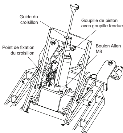
Figure 2 : Assemblage du vérin hydraulique
