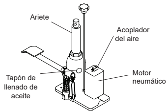
Unidad hidráulica operada por aire
