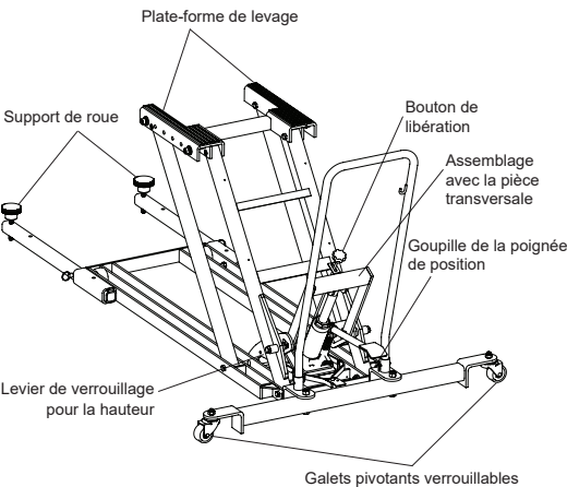
Figure 1 : Pièces des lève-tondeuses T-1250
