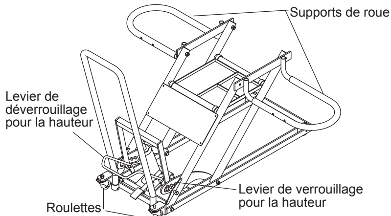
Figure 1 : Nomenclature du cric de levage
