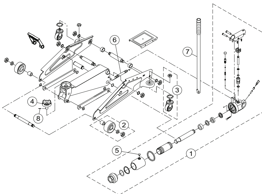
Figura 3 – Ilustración de las Partes de Repuesto
