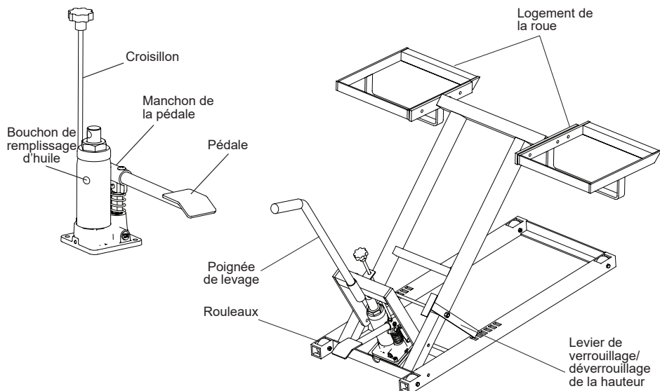
Nomenclature du cric de levage
