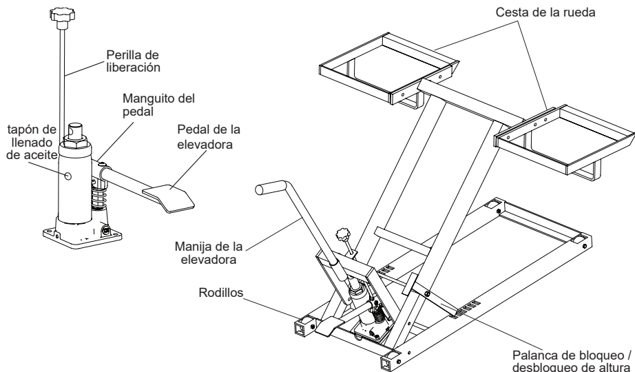
Nomenclatura de la elevadora para podadoras
