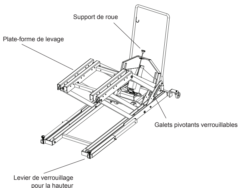
Figure 1 : Pièces des lève-tondeuses 2830425
