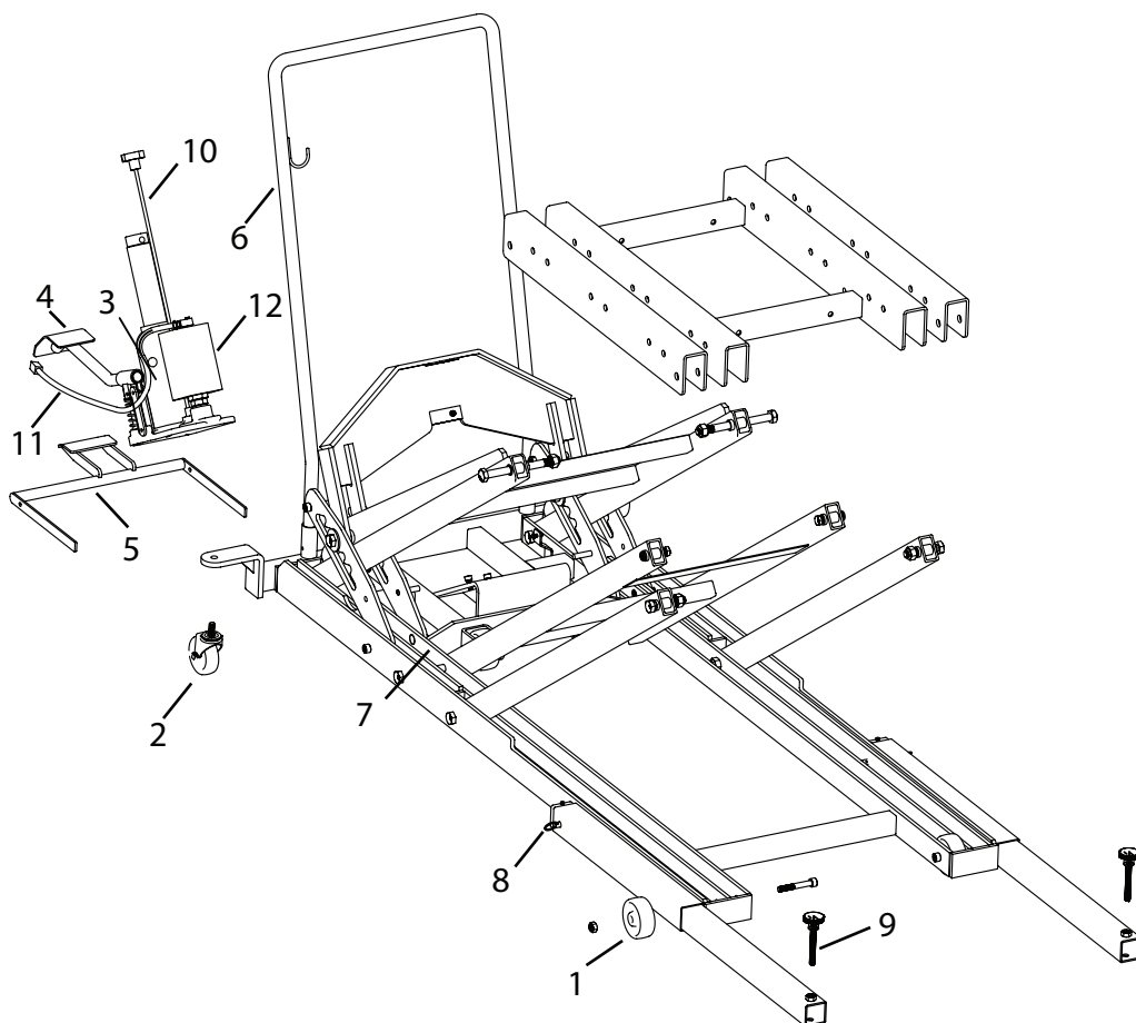
Figura 5: ilustración de piezas de repuesto para el modelo 2830425
