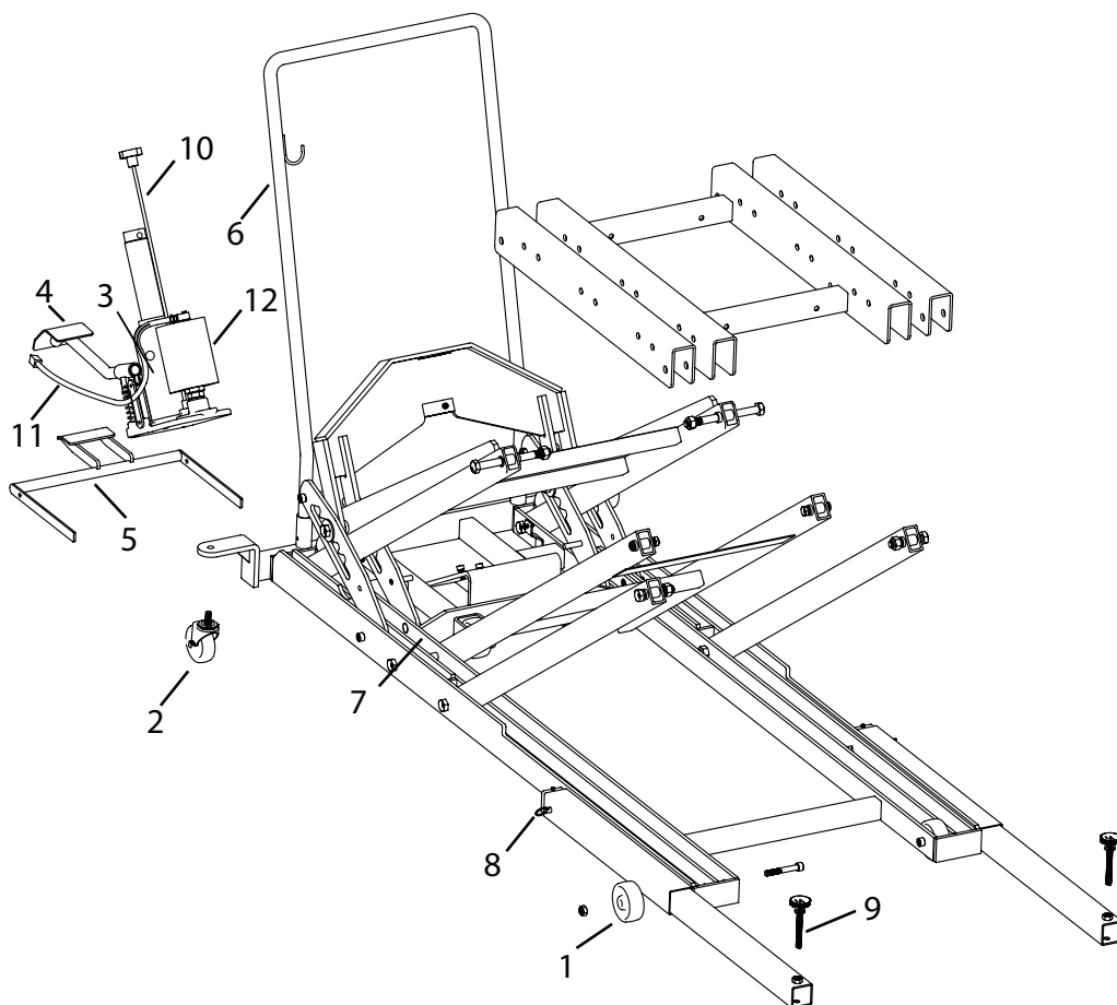
Figure 5 : Illustration des pièces de rechange du modèle 2830425
