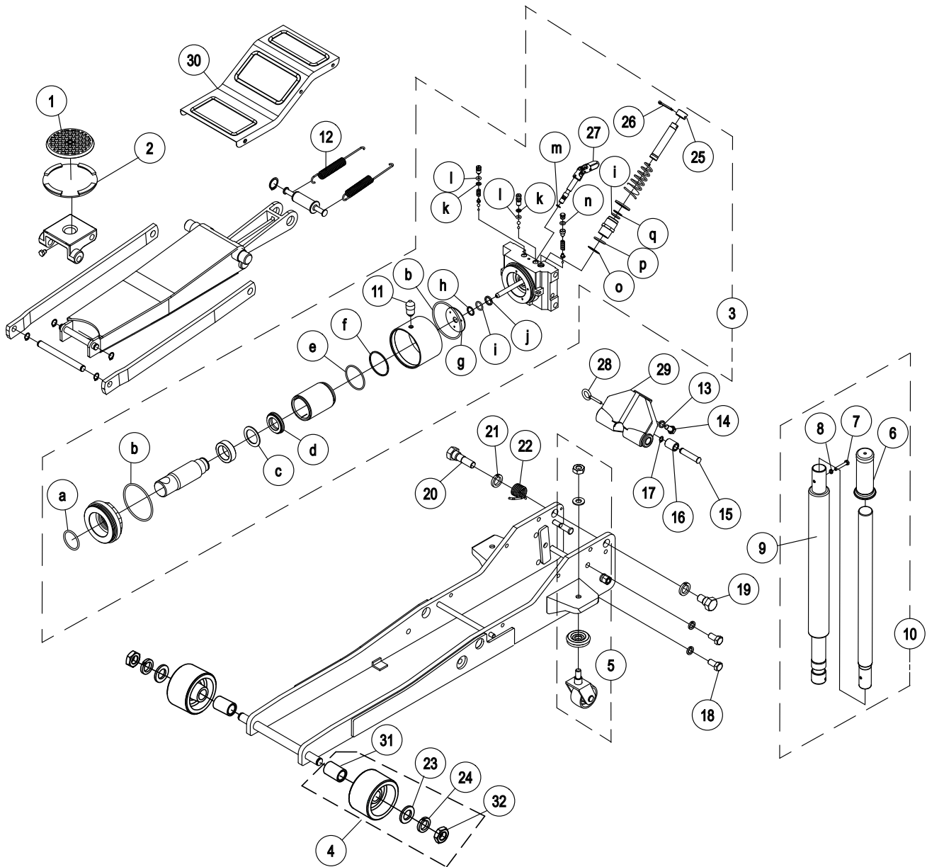
Figura 2: Ilustración de piezas de repuesto para el modelo 29023B
