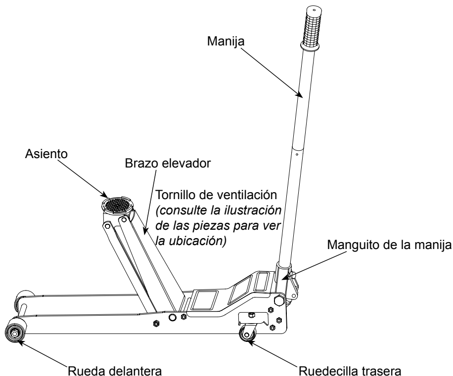
Figura 1: Nomenclatura del gato de servicio
