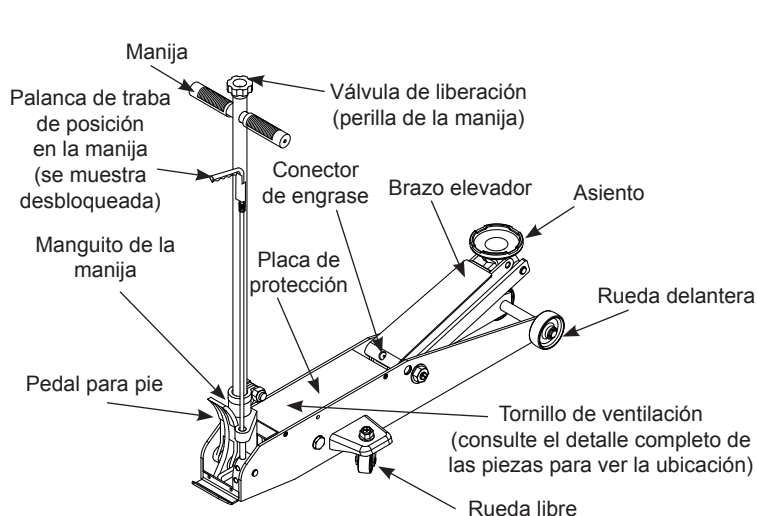
Figura 1: Componentes del modelo 25048C
