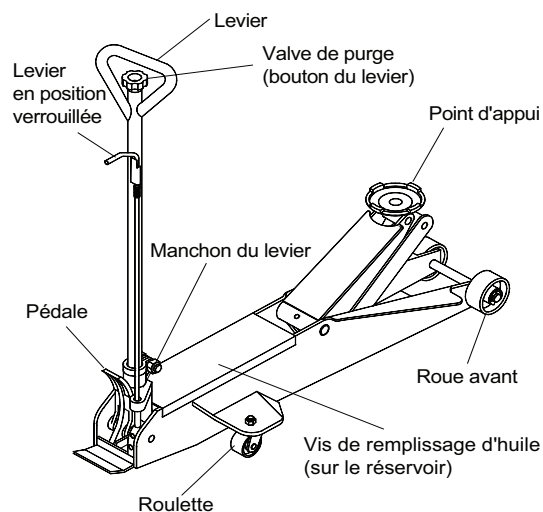
Figure 2 : Composants des modèles 25057 et 25107
