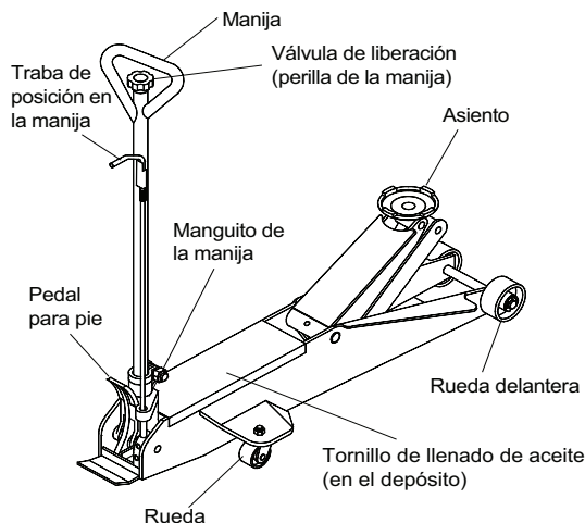
Figura 2: Componentes de los modelos 25057 y 25107
