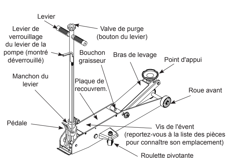
Figure 1 : Composants du modèle 25048C
