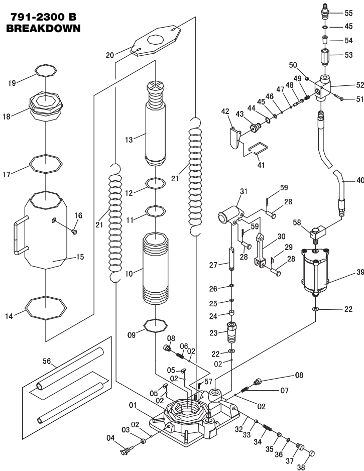
791-2320 B BREAKDOWN
