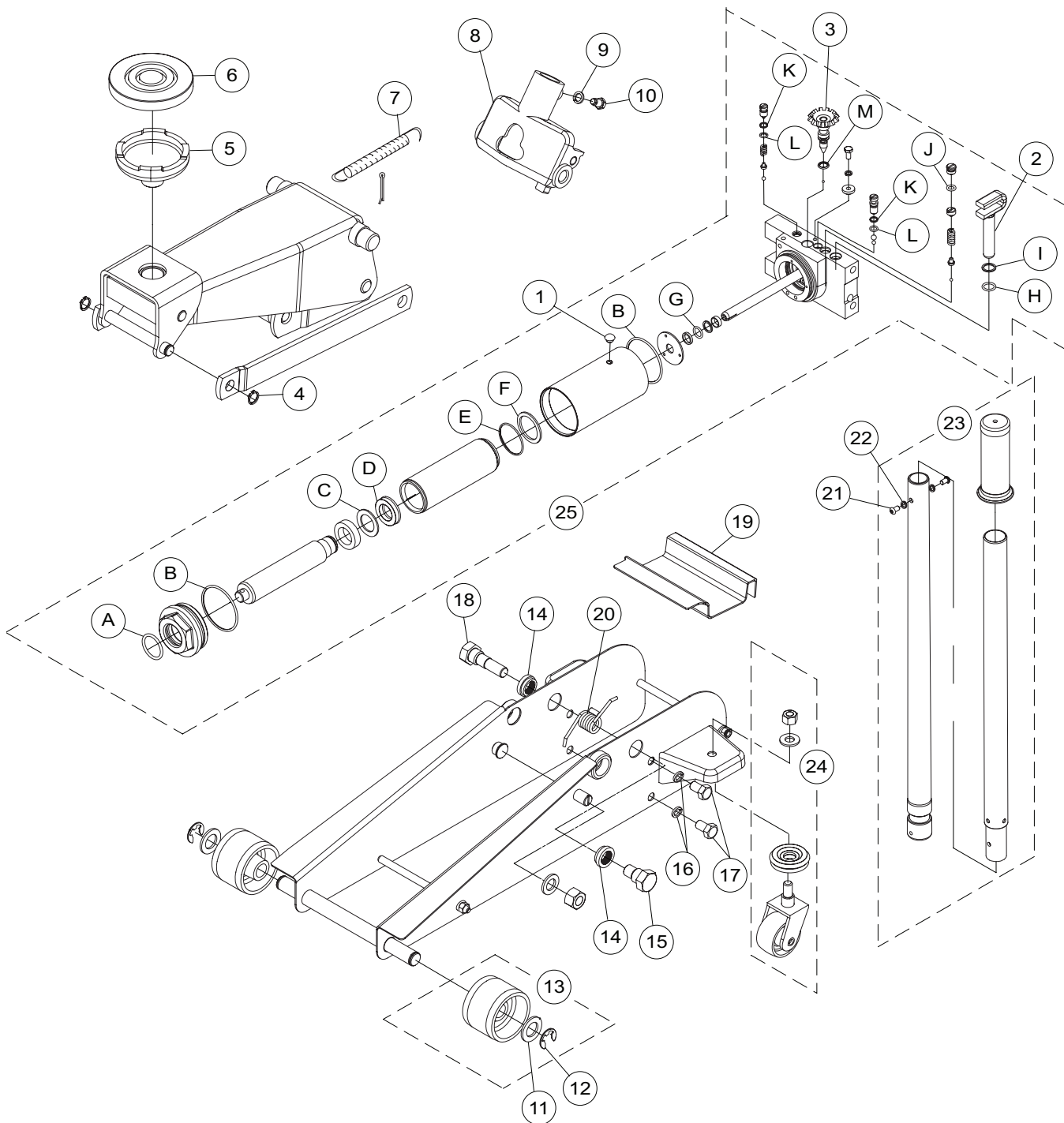
Figura 2: Ilustración de piezas de repuesto para el modelo MFJ3T
