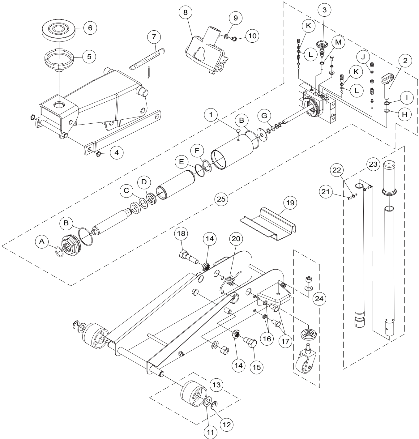
Figure 2 : Illustration des pièces de rechange du modèle MFJ3T
