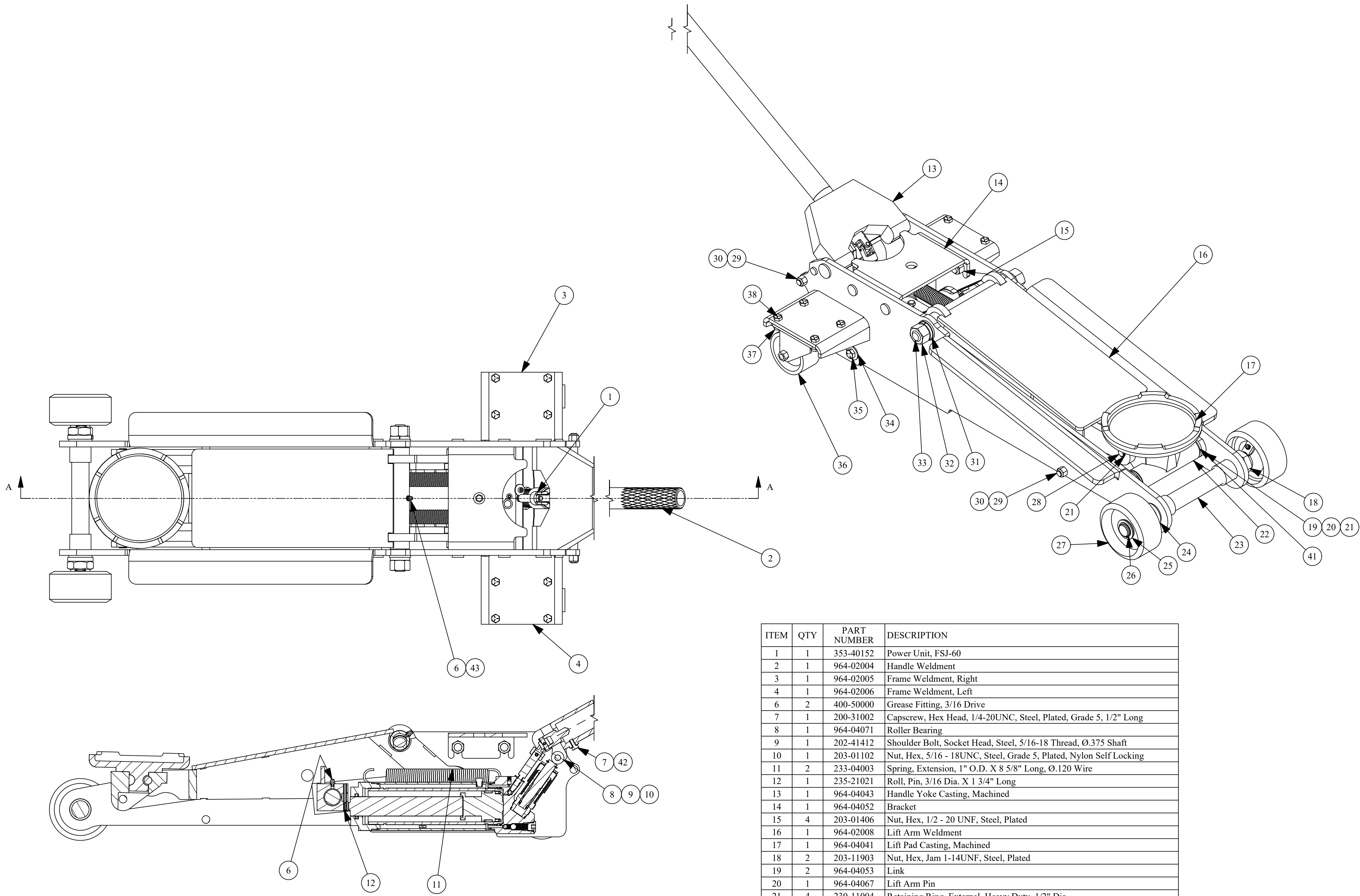
SECTION A-A SCALE 1:4
