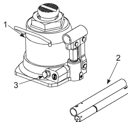
Figura 4: Ilustración para los modelos 5100767 y 5100769
