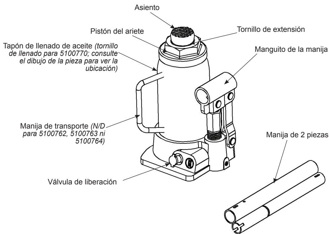
Figura 1: Nomenclatura habitual de un gato de botella (se muestra 5100768)
