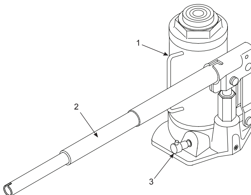
Figura 5: Ilustración para el modelo 5100770
