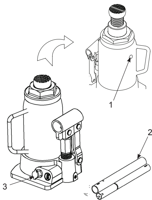
Figura 3: Ilustración para los modelos 5100765, 5100766 y 5100768
