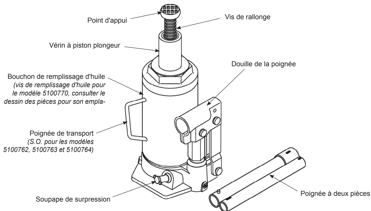
Figure 1 : Pièces d'un cric-bouteille typique (modèle 5100768)
