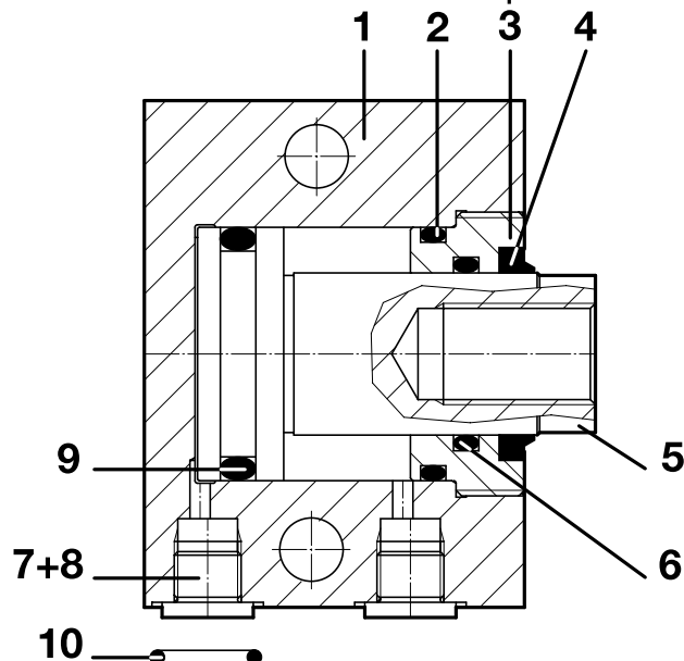
BD & BMD
