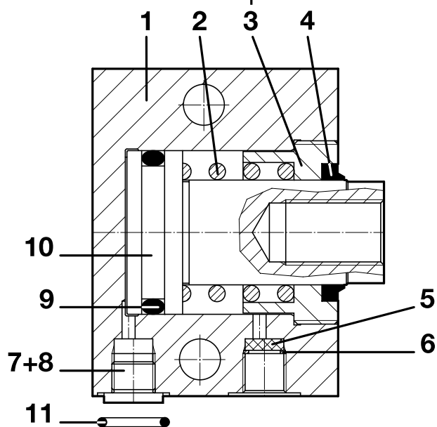
BS & BMS
