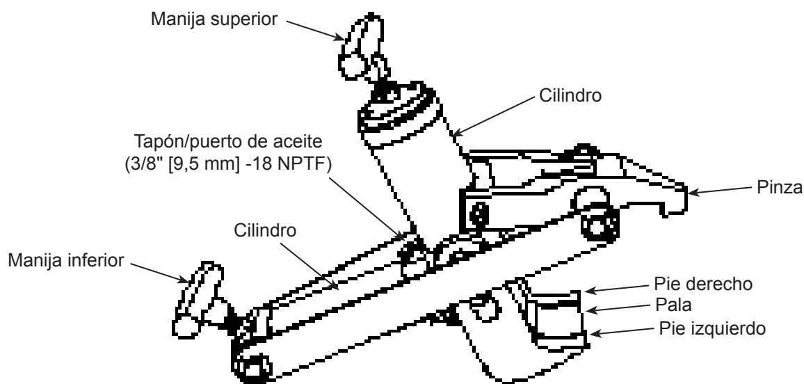
Figura 1: Componentes del modelo J22910
