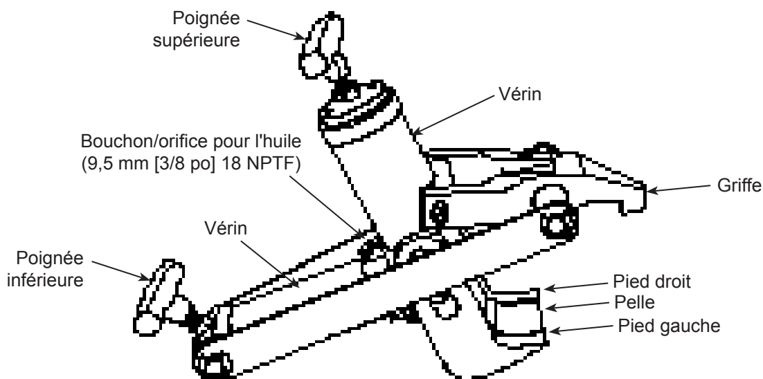
Figure 1 : Composants du modèle J22910
