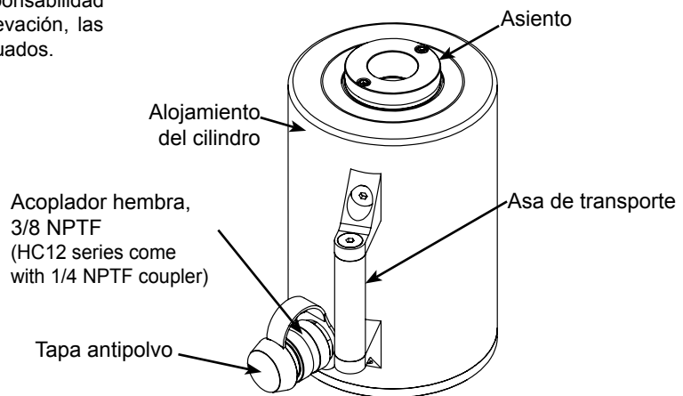
Figura 1: Componentes habituales del cilindro
