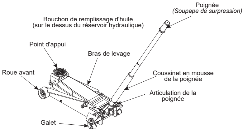
Figure 1 - Nomenclature typique de Jack
