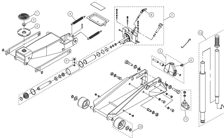
Figure 2 - Illustration des pièces de rechange pour le modèle B6350
